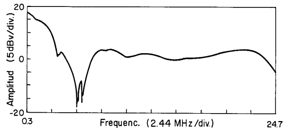
Figura 4. Alteración del espectro de Fig. 1, causada por un palpador END de 1 MHz.
