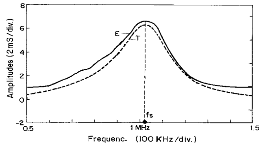
Fig. 5. Conductancia del transductor de carga de 1 MHz ( T = Teórica, E = Experimental ).
