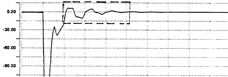
Fig. 7. Detalle del segmento inicial de un pulso excitador, reflejando alteraciones procedentes de la rama mecánica del palpador, y asociadas a la propia vibración pulsada del mismo.
