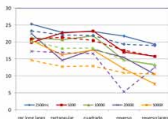
Figura n°8. Valores medios entre los 10 receptores de T_s en ms (izquierda) y de LF en % (derecha) en iglesias de diferentes formas y volúmenes con la fuente sonora en la posición A (—) y en D (---)
