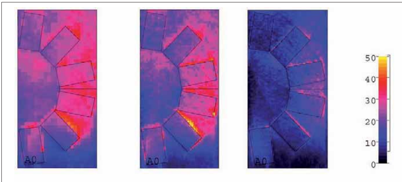
Figura nº5. Mapa en colores del parámetro LF (%) a 500 Hz, para el volumen de 2500 m 3 (izquierda, 1:400), 10000 m 3 (centro, 1:650) y 50000 m 3 (derecha, 1:1000) en iglesias de planta rectangular reverso largo con la fuente sonora en posición C
