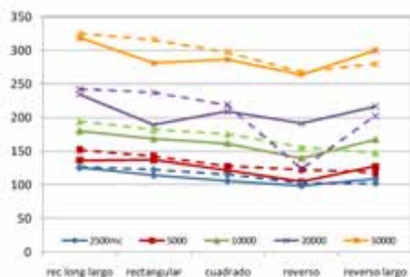
Figura n°8. Valores medios entre los 10 receptores de T_s en ms (izquierda) y de LF en % (derecha) en iglesias de diferentes formas y volúmenes con la fuente sonora en la posición A (—) y en D (---)
